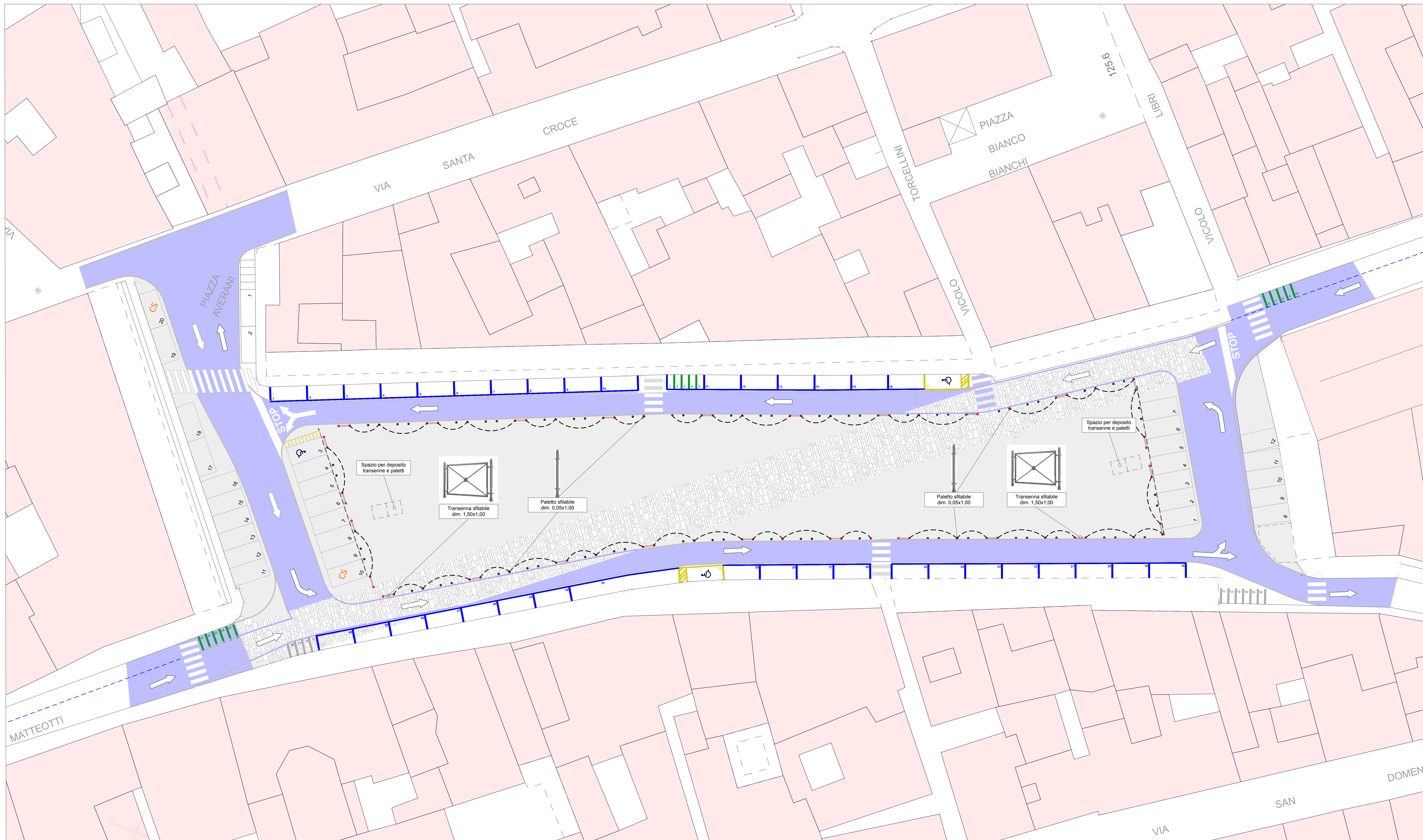
VIABILITÀ IN PIAZZA MARSILIO FICINO durante i lavori di rifacimento dei marciapiedi nei corsi Matteotti e Mazzini - Scala 1:200
